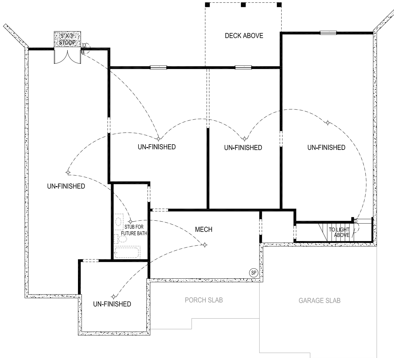
OPTIONAL BASEMENT
